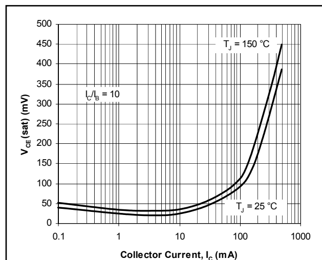
Fig. 3. V_{CE}(\text{sat}) vs. I_C
